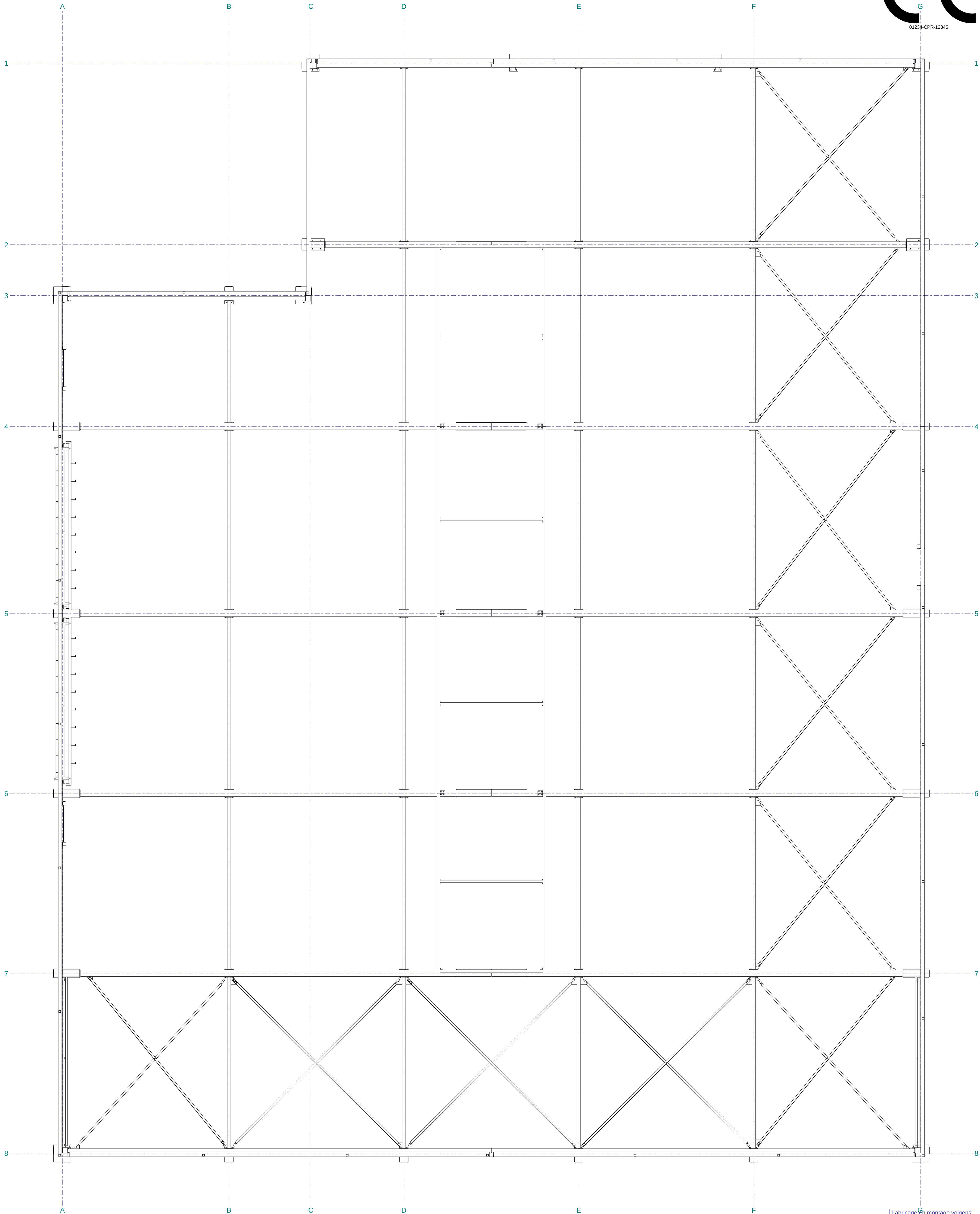
3d - enkel staal 1:50
